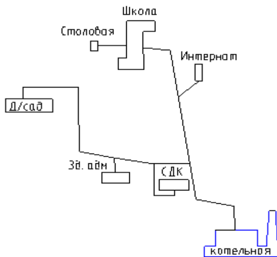
Рис. 2.3.1. Схема тепловой сети котельной села Самсоново
